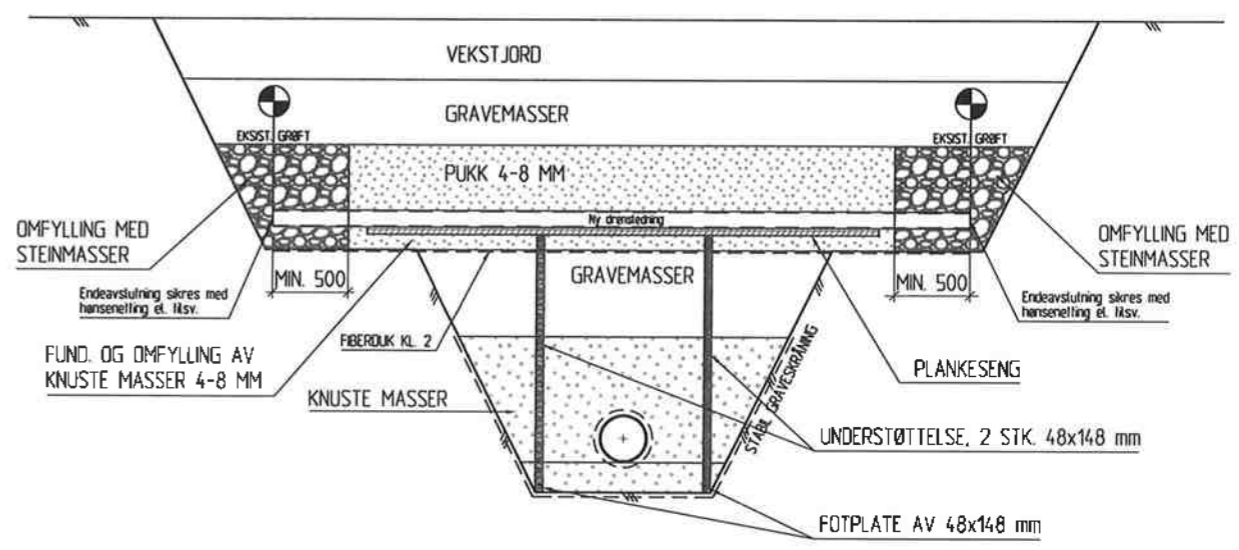
LØSNING VED STEINSATT DRENSGRØFT VED DYPE GRØFTER
