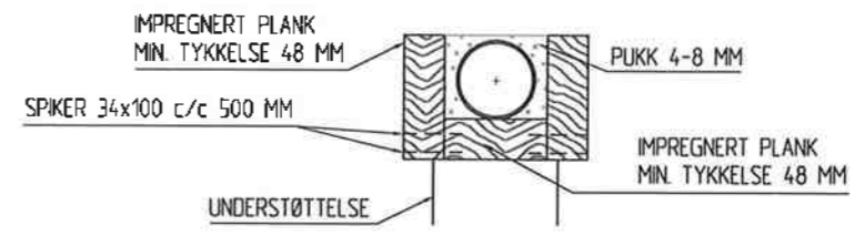
DETALJ AV PLANKESENG
