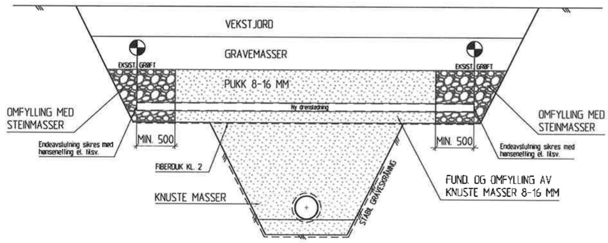
LØSNING VED STEINSATT DRENSGRØFT MED OPPFYLING MED PUKK
