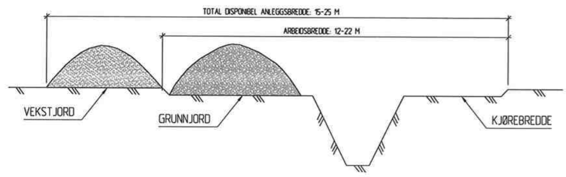
DISPONIBEL TRASEBREDDE OVER DYRKET MARK; GENERELT SNITT
