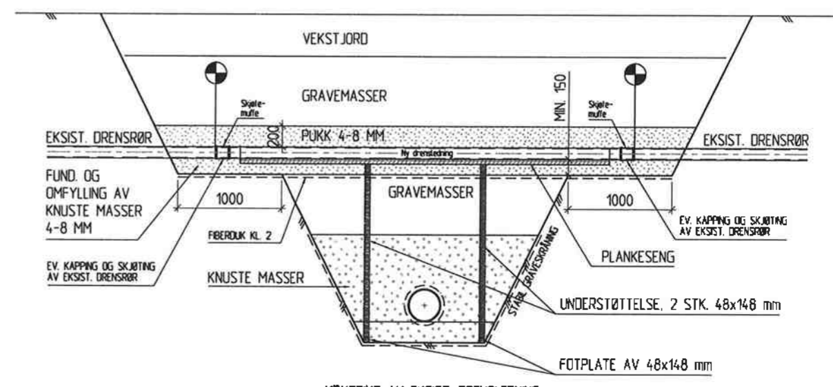
KRYSSING AV EKSIST. DRENSLEDNING VED DYPE GRØFTER
